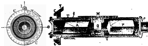
Fig. 2. — Lunette Mesuré et Nouel.
